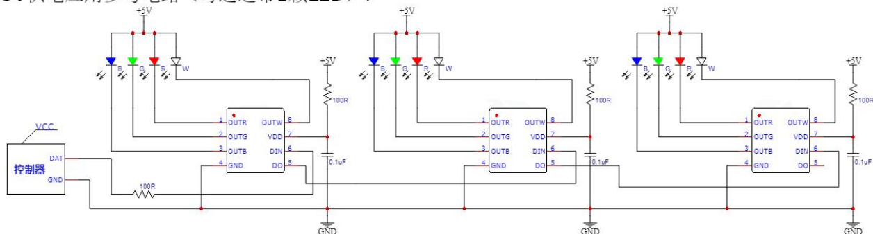
2. 12V供电应用参考电路（每通道带3颗LED）：
