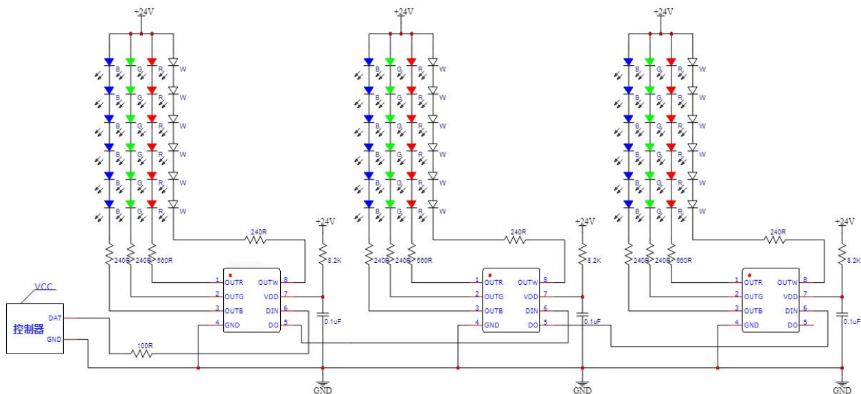
3. 24V供电应用参考电路（每通道带6颗LED）：
